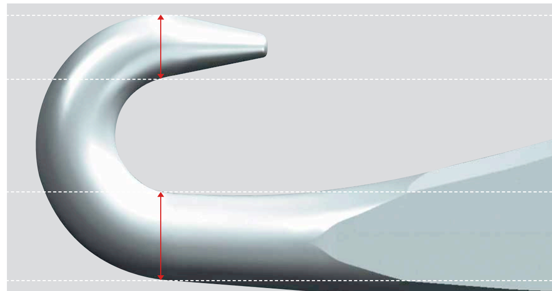
锥形针钩: 减少横截面面积以增加纱线活动空间(见上方箭头), 增加横截面面积来优化针钩的稳定性(见下方箭头)
